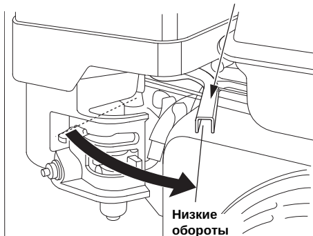
РЫЧАГ УПРАВЛЕНИЯ ДРОССЕЛЬНОЙ ЗАСЛОНКОЙ
