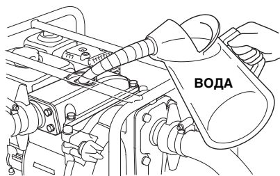
ПРОБКА ГОРЛОВИНЫ ВОДЫ ДЛЯ ПРЕДВАРИТЕЛЬНОЙ ПРОКАЧКИ
