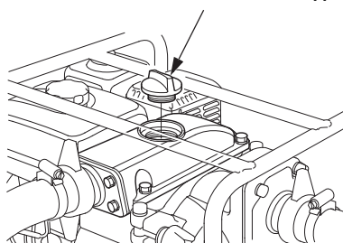
ПРОБКА ГОРЛОВИНЫ ВОДЫ ДЛЯ ПРЕДВАРИТЕЛЬНОЙ ПРОКАЧКИ
