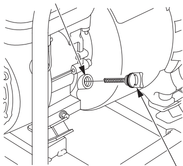
ПРОБКА МАСЛОСЛИВНОЙ ГОРЛОВИНЫ / МАСЛЯНЫЙ ЩУП
